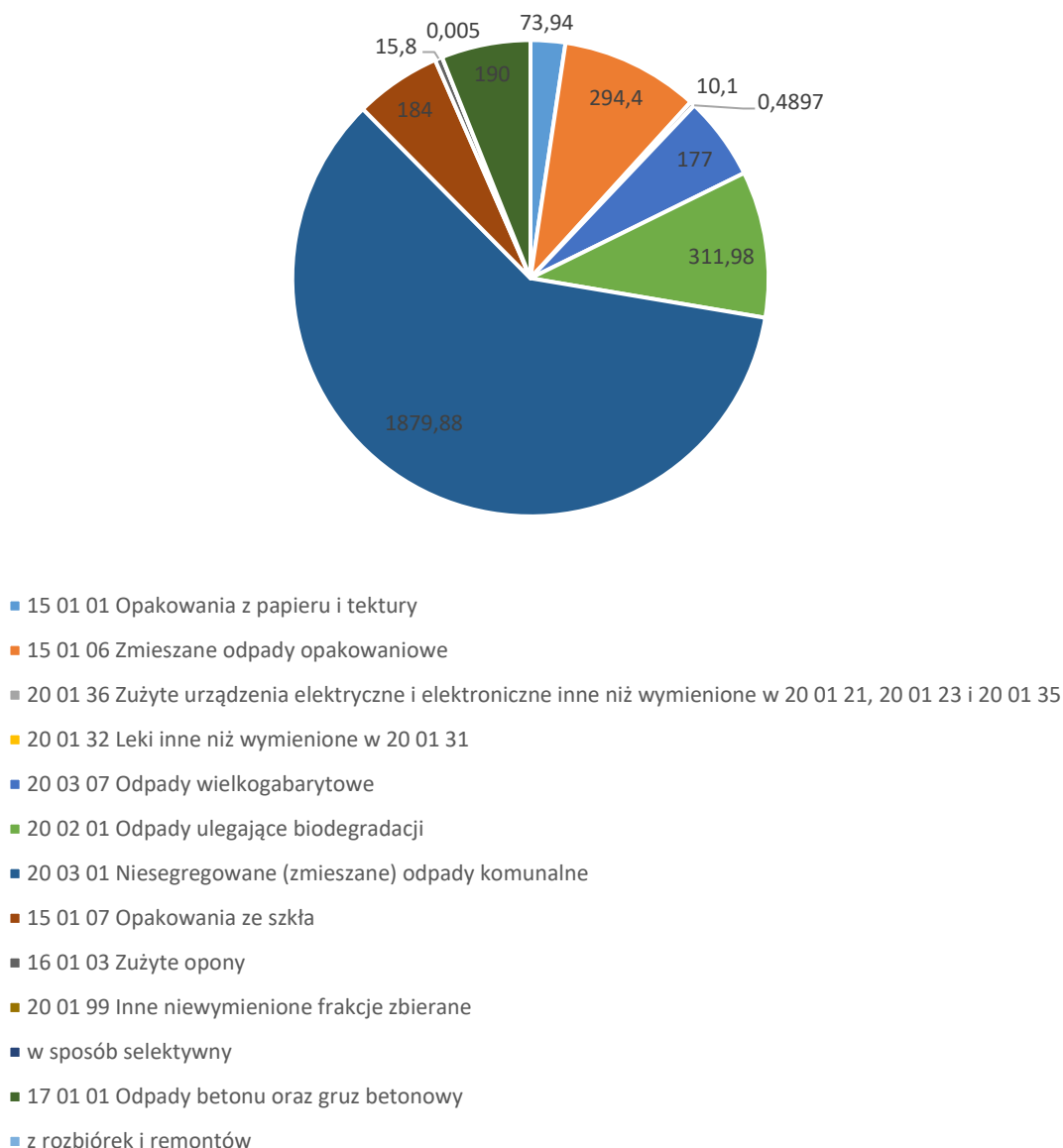
Rodzaje i ilości wytwarzanych odpadów w 2021 roku
